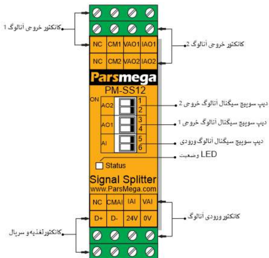
نمای اتصالات
